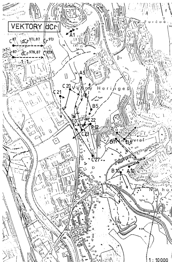
Obr.4. Vektory redukovaných diferencií dCr zo súradníc C^{87} a Cr^{97J} , Cr^{97N} .
