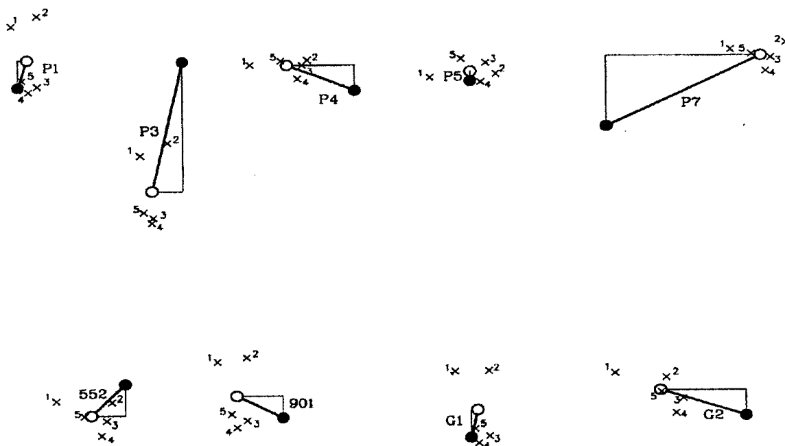
Obr. 3: Rozpory medzi polohami C^J a C^{Jto} M - polohy bodov - 1:1, ● – katastrálna súradnicová poloha, x – z GPS meraní určená súradnicová poloha, ○ – z GPS meraní určená priemerná súradnicová poloha Fig. 3: Discrepancies among C^J C^{Jt} and C^{Jto} positions
