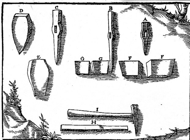
Obr. 2. Želízko A-zasekáček, B-želízko žumpové, C-skální klín, D-klín, E-hrubý klín, F-plechový klín, G-dřevěná rukojeť H-v želízku zasazená rukojeť.
