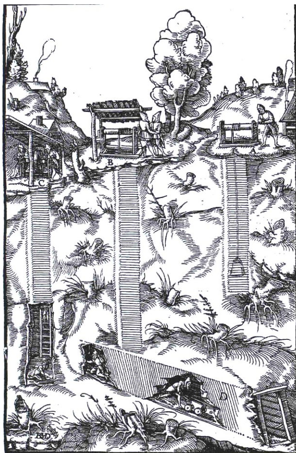
Obr. 3. Tři svislé šachty, z nichž první ještě nedosahuje ke štole A. Druhá šachta B dosahuje ke štole. K třetí ještě štola nedošla C. Štola D.
