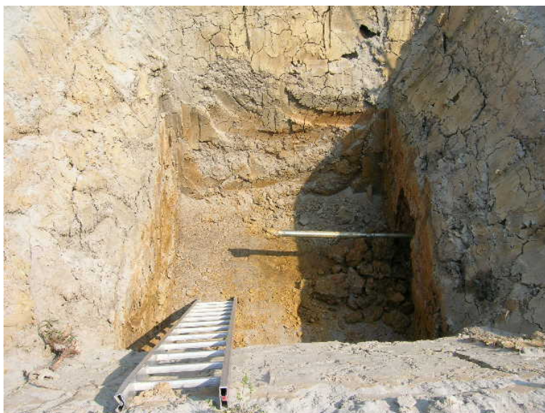
Abb. 11. Blick in die Zielgrube der ersten Erdsonden-Bohrung. Der Horizontalbohrkopf ist exakt im Zielbereich angekommen (Stuttgart-Vaihingen). Fig. 11. The drill head reached exactly the planned trace in the aim pit.
