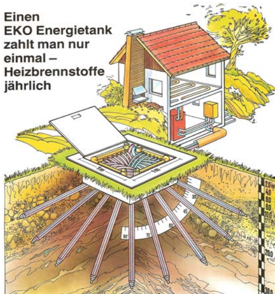
Abb. 1. Einen EKO Energietank zahlt man nur einmal – Heizbrennstoffe jährlich. Fig. 1. The Tracto-Technik-ECOTHERM-Method (figure from 1984) for a geothermal utilisation with the percussion tool ramming of steel pipes in a radial arrangement to the ground.
