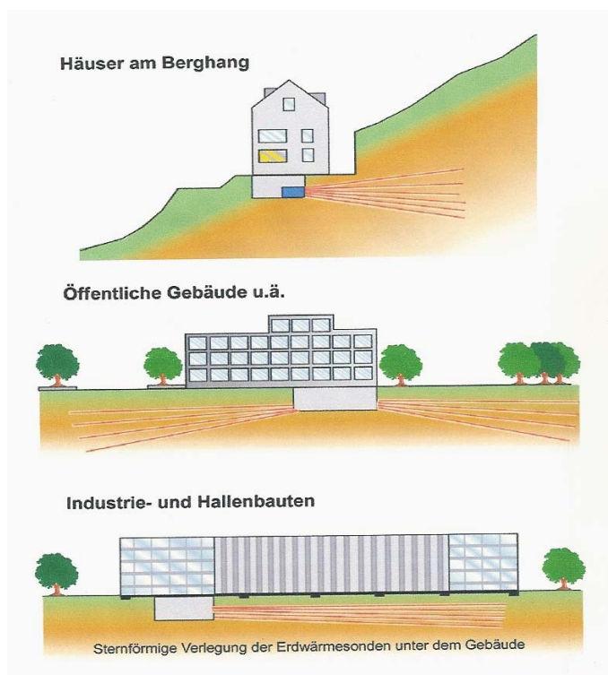
Abb. 16. Kostengünstige Erdwärmeerschließung mit TT-Bohrgeräten – Einsatz von GRUNDOPIT – Geräten. Fig. 16. Examples for the application of horizontal sond layings with the TT drilling machines.
