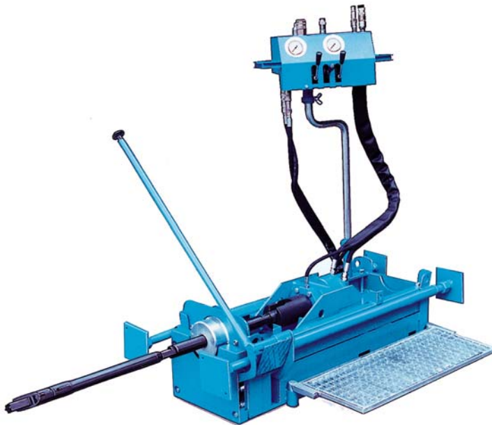
Abb. 7. Das Basisgerät für ein kostengünstiges und schnelles Geothermie-Bohrgerät: GRUNDOPIT von Tracto-Technik.
