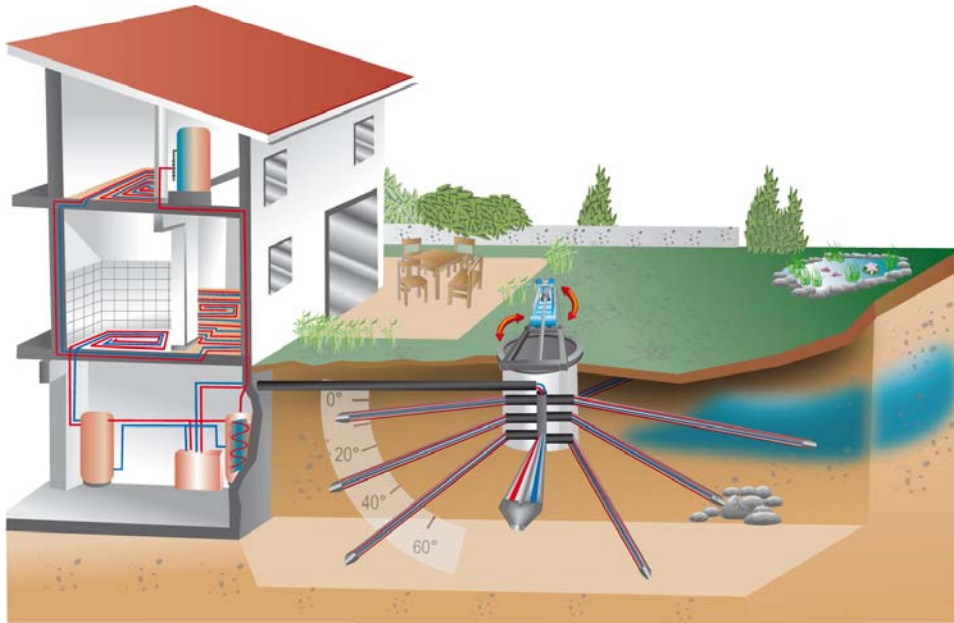
Abb. 2. Das neue Geothermal Radial Drilling von TRACTO-TECHNIK greift auf frühere gute Erfahrungen zurück. Fig. 2. The new Geothermal Radial Drilling (GRD-) method by Tracto-Technik.
